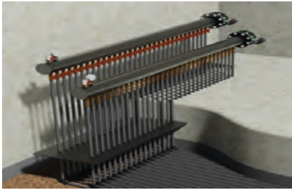
Schnittdarstellung des Systems mit aufgebauter Verteilereinheit
