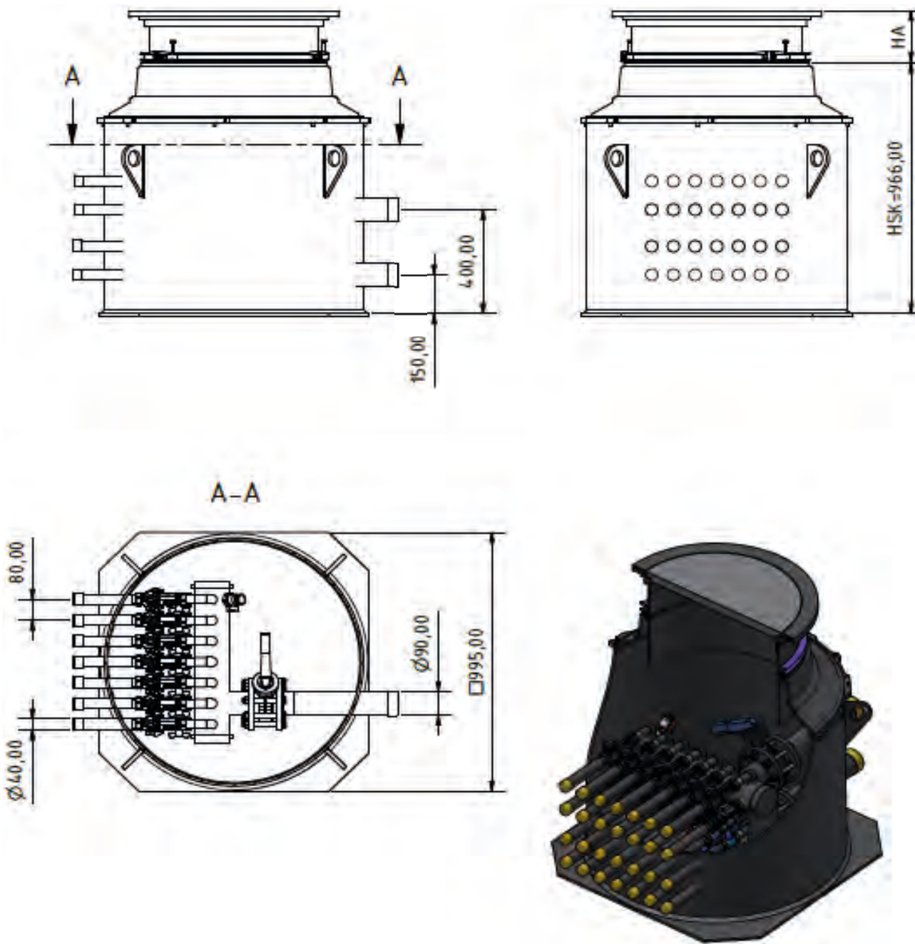
Innendurchmesser Schacht: 940mm Bis 10 Fach auch einreihig ausführbar
