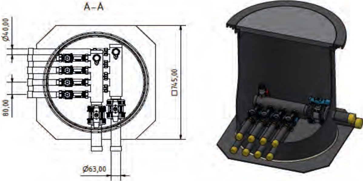
Innendurchmesser Schacht: 612mm
