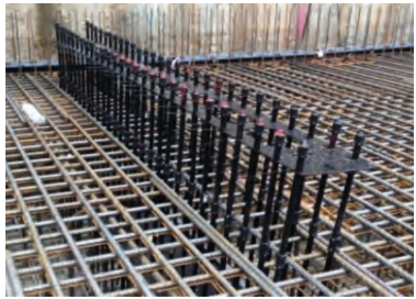
Systemaufbau in der Bewehrung mit zus. Führungsplatte für die Abstandsfixierung der Durchgangsrohre
